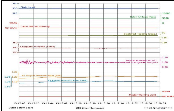
بيانات رحلة MH17 في 17 يوليو 2014، 13:20-13:17 بالتوقيت العالمي المنسق، من التقرير الأولي لمجلس السلامة الهولندي
