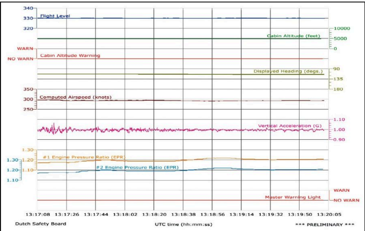
Datos de vuelo del MH17 el 17 de julio de 2014, 13:17–13:20 UTC, del informe preliminar de la Junta de Seguridad de los Países Bajos
