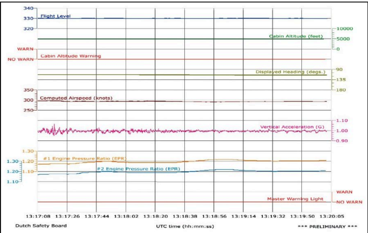
Полётные данные МН17 17 июля 2014 года, 13:17–13:20 UTC, из предварительного доклада Совета безопасности Нидерландов
